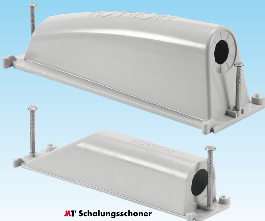
MT Schalungsschoner M20/M25/M32 E-No 126 588 063 grau
